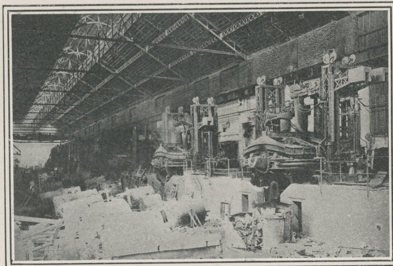
VUE DU HALL DES FOURS ÉLECTRIQUES PAUL GIROD
