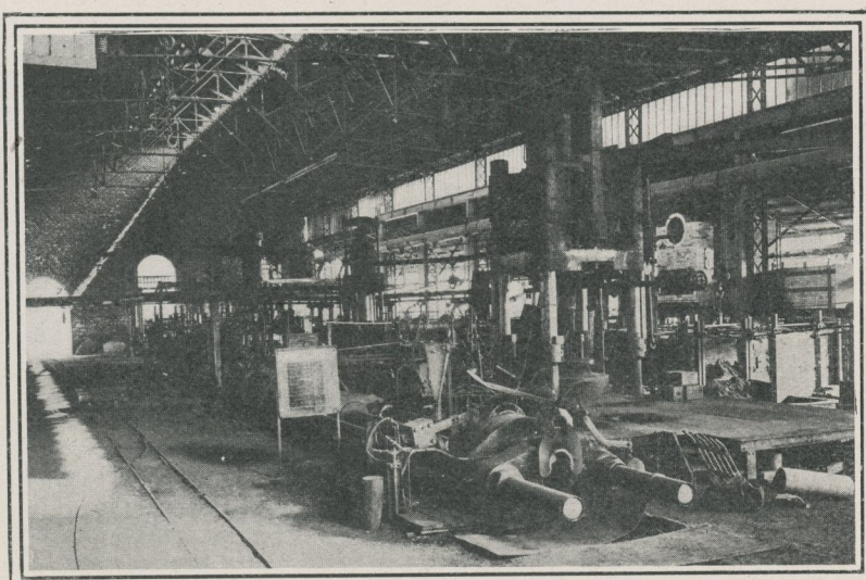
PRESSES A EMBOUTIR LES OBUS DE GROS CALIBRES AUX USINES PAUL GIROD
